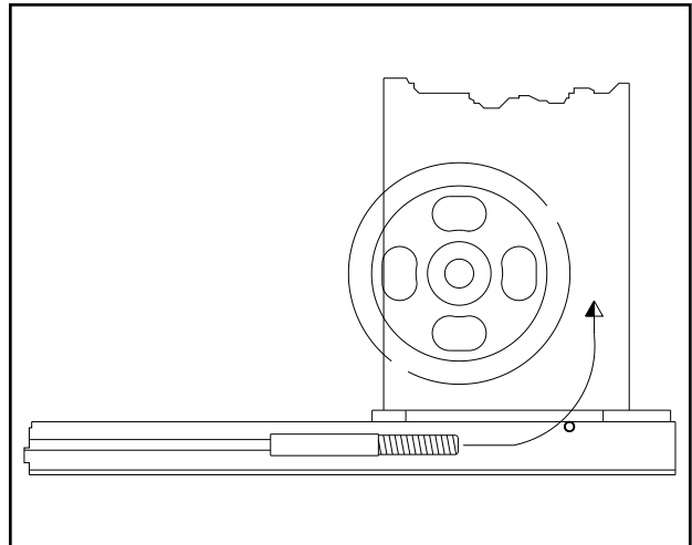
Fig.40 Inserimento del codulo filettato Fig.40 Inserting the threaded end
