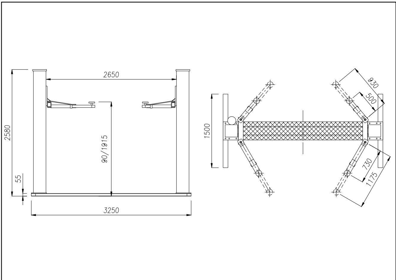
Fig.9 Dimensioni ed ingombri
