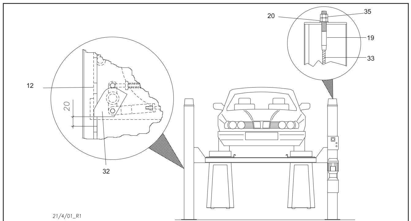
Fig.59 Registrazione funi
