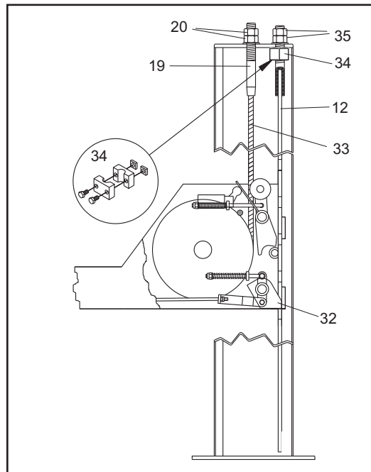
Fig.53 Preregistrazione funi
