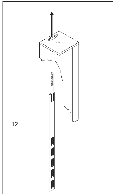
Fig.43 Sfilare l'asta di sicurezza dall'alto della colonna
