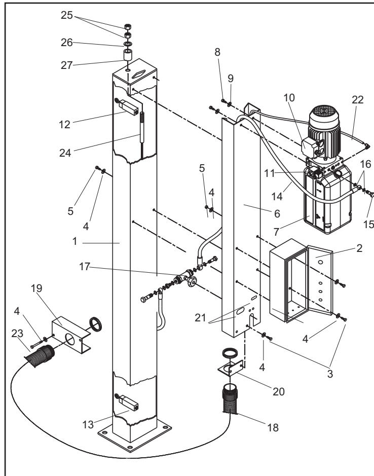
Fig.44 Preparazione colonna 1
