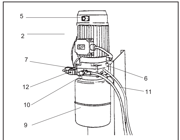
Fig.6A Centralina idraulica. Fig.6A Hydraulic power unit.
