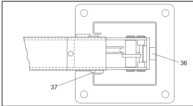
Fig.55 Regolazione pattini
