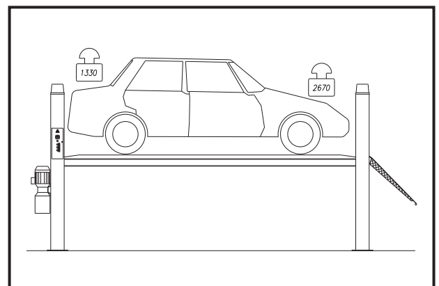
Fig.18 Ripartizione pesi "B" Abb.18 Lastverteilung "B"
