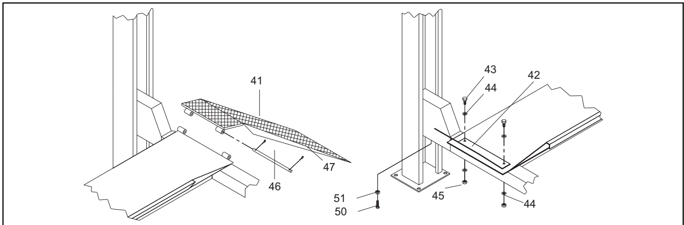
Abb.58 Fixierung der Auffahrampen und der Reifenblockiervorrichtung
