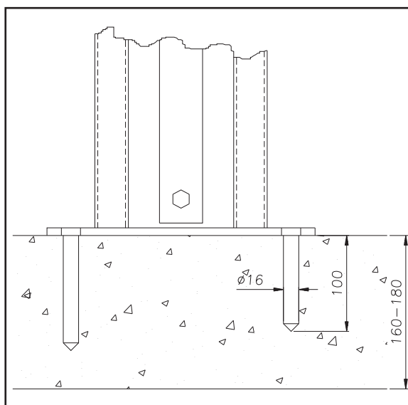
Abb.57 Fixierung der Säulen
