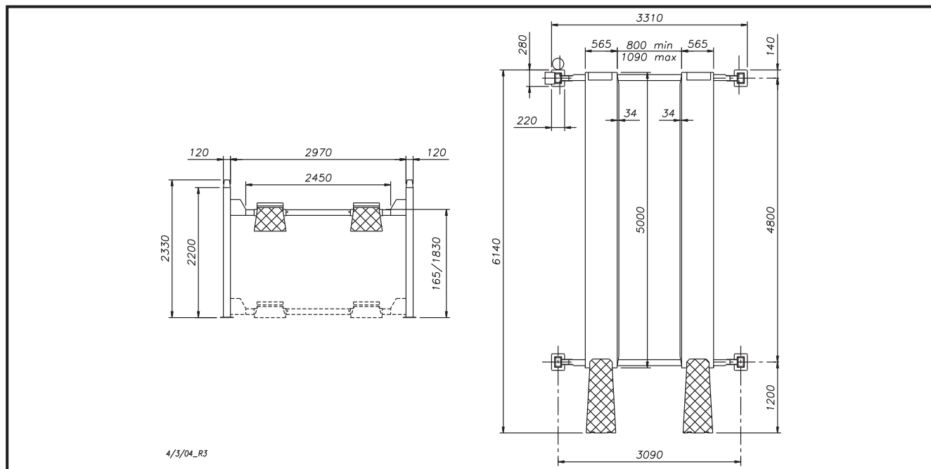
Fig.11 Dimensioni ed ingombri
