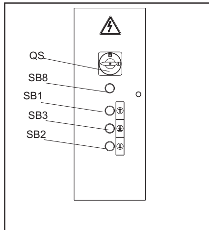
Fig.52 Pannello di comando Abb.52 Schaltfabel
