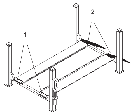
Abb.20 Verschiebung in der Länge mit Schutzmaßnahm
