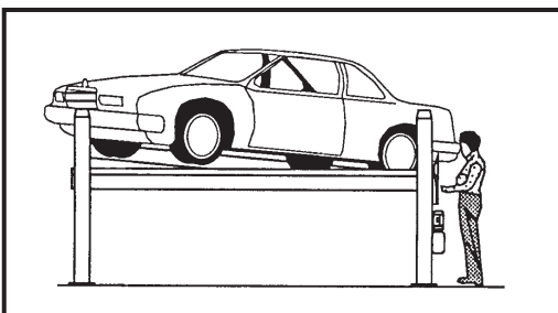
Fig.32 Rischio di caduta del veicolo
