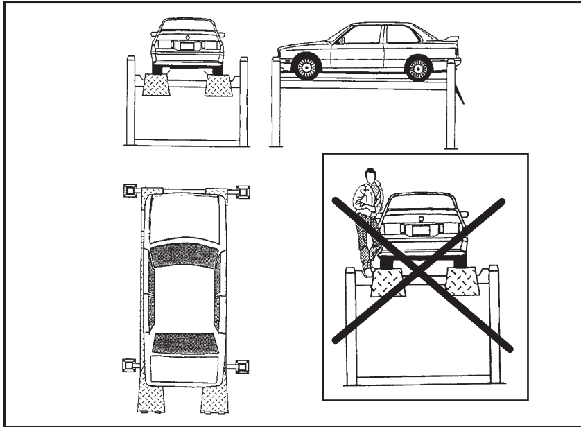
Fig.22 Veicolo caricato correttamente
