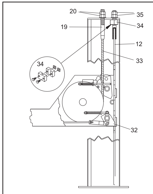
Fig.53 Preregistrazione funi Abb.53 Voreinstellung der seile
