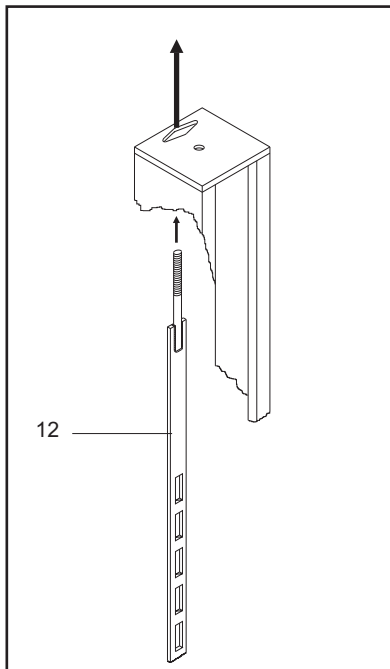
Abb.43 Vom obersten Punkt der Säule den Abschaltstab einführen
