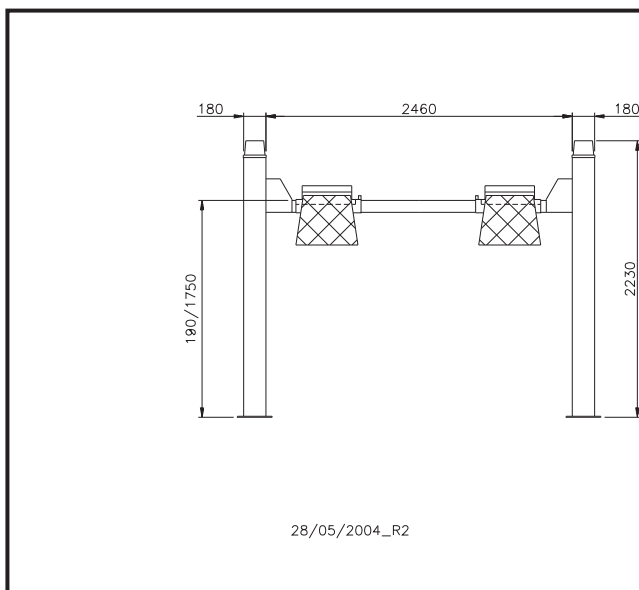
Fig.11a - Dimensioni ed ingombri con pedane senza incavo per assetto ruote
