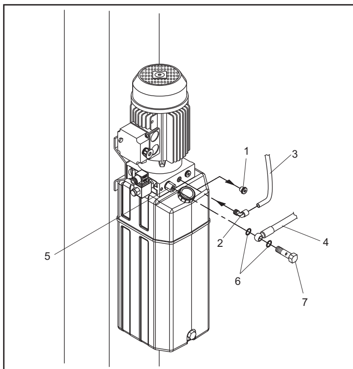
Fig.49 Allacciamento impianto idraulico
