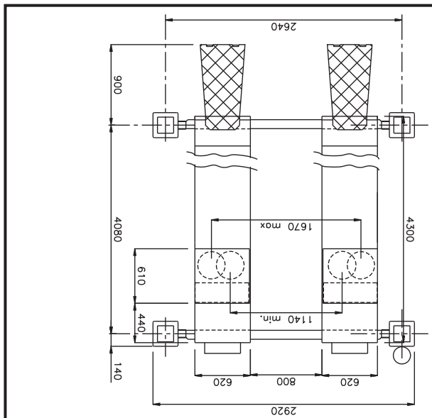
Fig.11 - Dimensioni ed ingombri con pedane per assetto ruote
