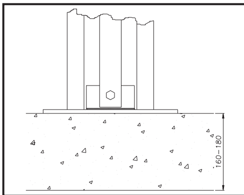
Fig.40 Spessore pavimentazione
